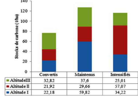
Figure 8 : Variation du stock moyen de carbone en fonction les catégories de système suivant le gradient altitudinal
